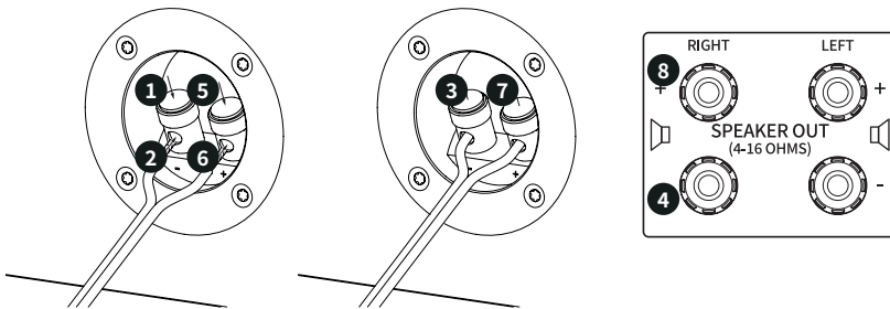
Abbildung 7. HM5 - Anschluss Lautsprecherkabel (ohne Stecker).
