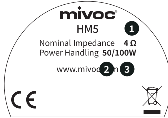
Abbildung 9. HM5 - Technische Angaben im Anschlussterminal.
