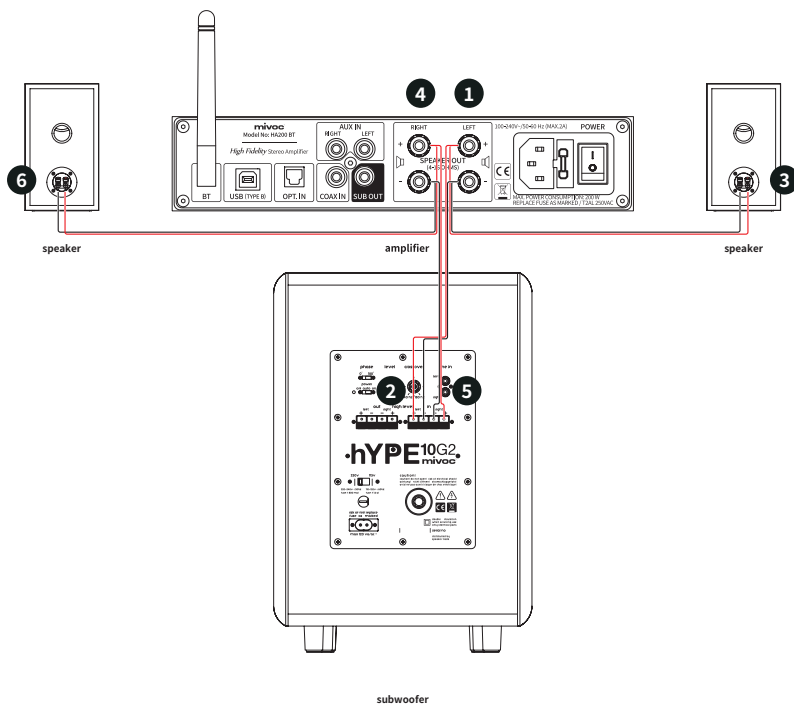
Figura 12. hYPE 10G2: conexión de audio con la entrada HIGH LEVEL.
