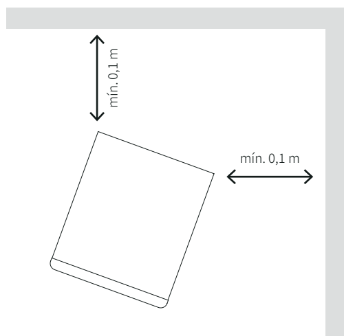
Figura 17. hYPE 10G2: distancia mínima respecto a las interfaces.
