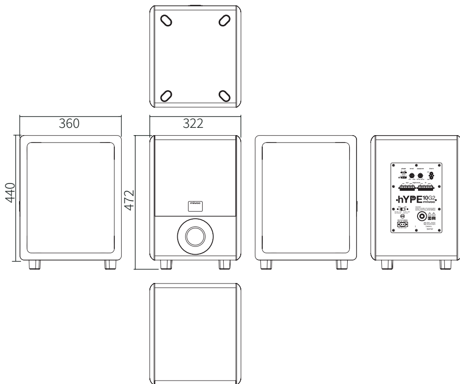
Figura 18. hYPE 10G2: dimensiones (mm).
